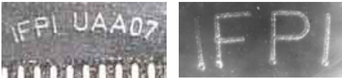
Рис. 13, 14. Код IFPI, виконаний за допомогою лазерного променя, на окантовці робочій поверхні «чистого» диска, що призначений для запису (рис. 13 — фотознімок з масштабною лінійкою, рис. 14 — зображення маркування зі збільшенням 21×)
