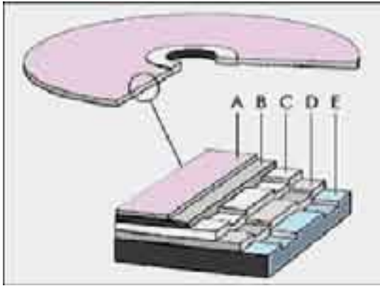
Рис. 11. Шари компакт-диску, призначеного для запису контрафактного примірника твору: А – шар поліграфічного зображення; В – захисний лак; С – відображуючий шар (алюмінієвий), D – активний шар для запису; E – основа (полікарбонат)
