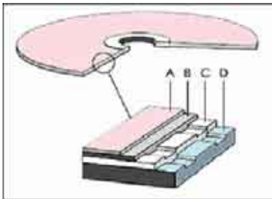
Рис. 12. Шари компакт-диску, виготовленого за технологією інжекційного лиття та призначеного для запису ліцензійного примірника твору: А – шар поліграфічного зображення; В – захисний лак; С – відображуючий шар, D – основа (полікарбонат) 1
