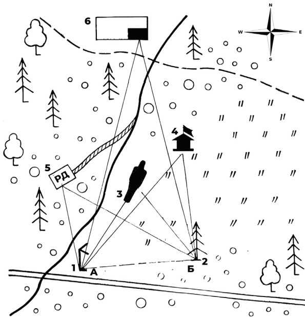
Рис. 140. План місцевості методом вимірювань за спрямованістю або за способом засічок: А – вихідна точка; Б – перший з об'єктів, що наноситься на план; 1, 2, 3, 4, 5, 6 – об'єкти, на які проводилося візування з точок А і Б; РД – речові докази
