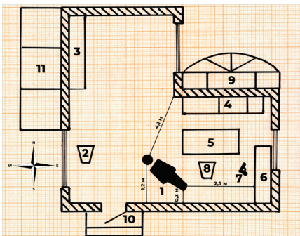
Рис. 137. Схематичний площинний план кімнати
